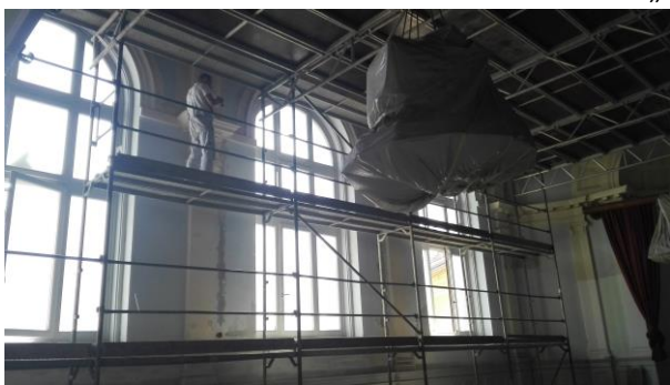
Teherbírási növelő „öszvér” szerkezet betonozás előtt
